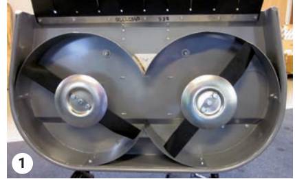
Angekipptes Mähwerk
