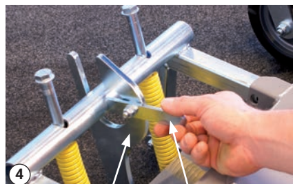
Verriegelung Griff
