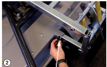
Verriegelung
